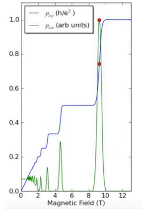
Obr. 10: Závislosť odporu od magnetickej indukcie 14
