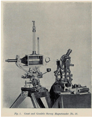
Obr. 11: Zememeračský magnetometer 15
