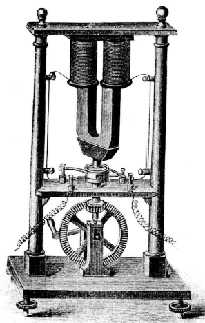
Obr. 3: Dynamo Hippolyta Pixiho – magnet tvaru U otáčame klukou pod dvojicou cievok 5
