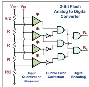
Obr. 8: Schéma flash ADC prevodníka 11
