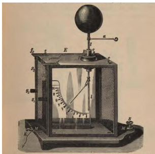
Obr. 1: Kolbeho elektrometer – ručička prístroja je vychylovaná elektrostatickým pôsobením 1
